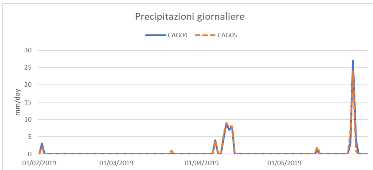
Grafico 3: precipitazioni giornaliere
